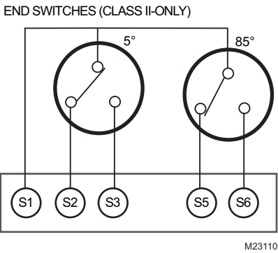
Fig. 13. End switches
